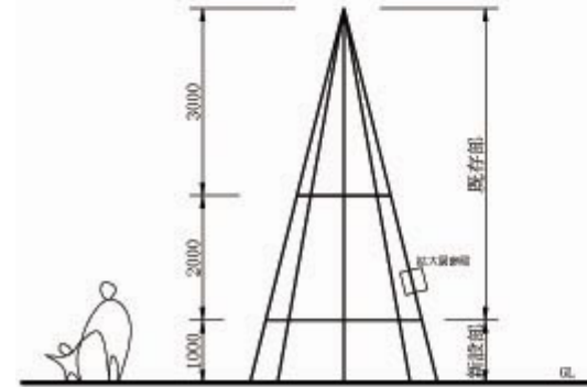
正面図 1:50
