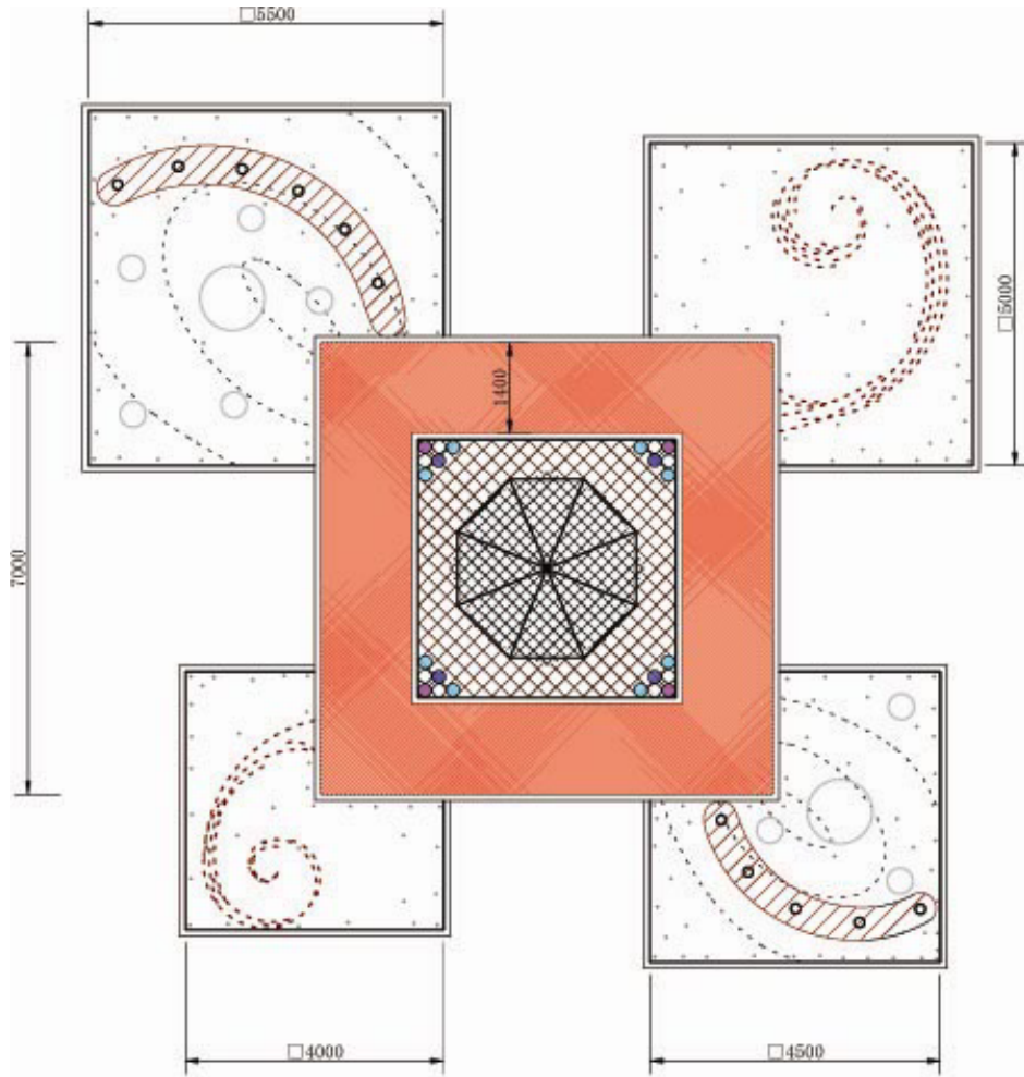
平面図 1:100
